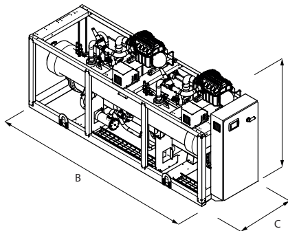
WTX 1300 - 2350
