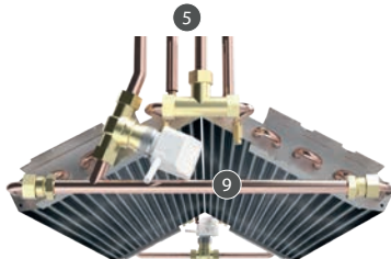
Hydraulische Anschlüsse und Steuerungskomponenten auf der Hydronikseite (zwei 2-Wege-Ventile und Stellantriebe im Inneren des Endgeräts).
